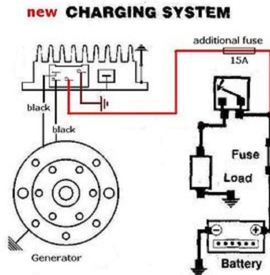
neue Verkabelung
