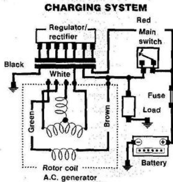
original Verkabelung
